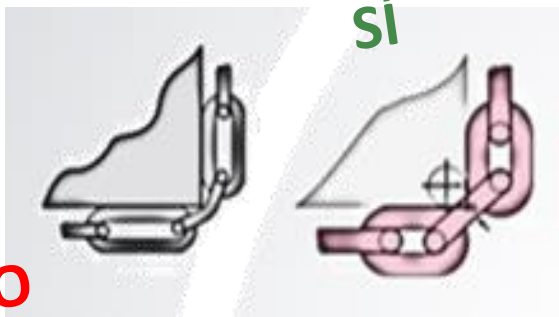
Imágenes extraídas de la norma UNE-EN 818. Cadenas de elevación corto. Seguridad. Eslingas de cadena.
